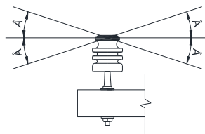
Figura 8 – Ângulo de deflexão vertical do primário rede nua (convencional)
